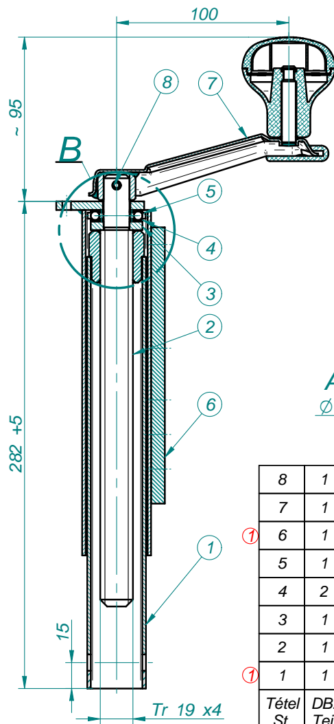
Metszet A-A
