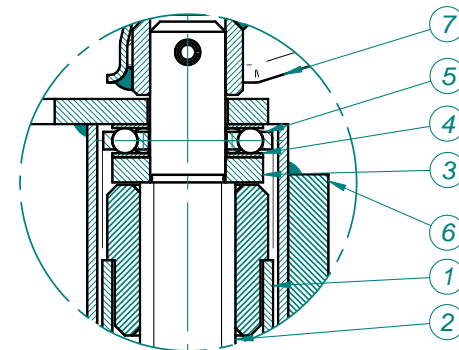
Részlet B 1:1
